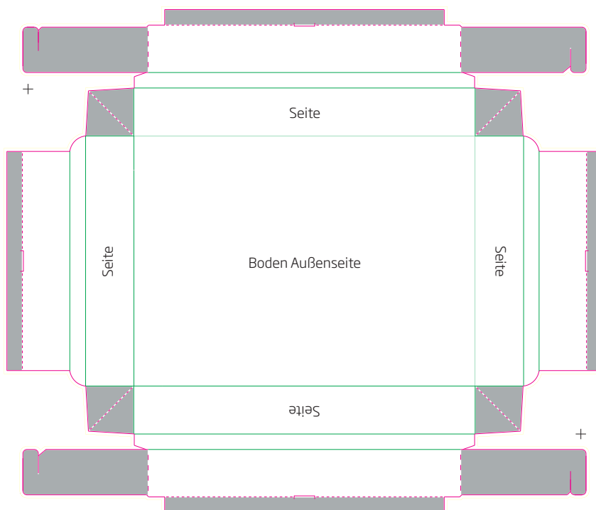
Unterteil
